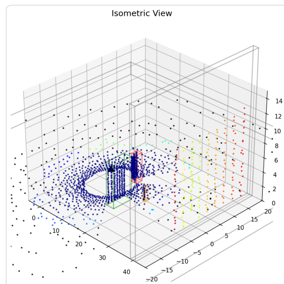
等轴视图
