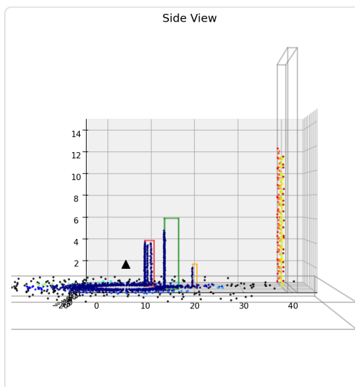
侧视图
